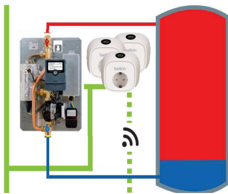
Pufferspeicher mit Schichtenbeladung
