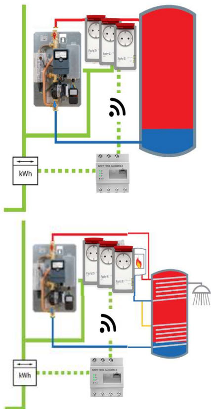
Pufferspeicher mit Schichtenbelastung
